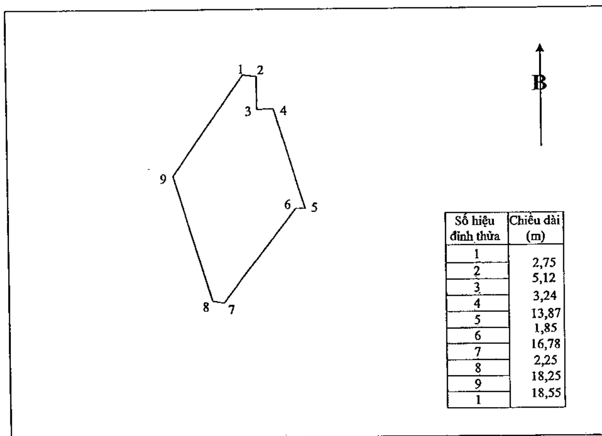
Hình 2. Sơ đồ thửa đất có nhiều cạnh thửa
